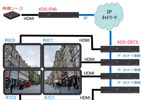
2x2ビデオウォール構成例
