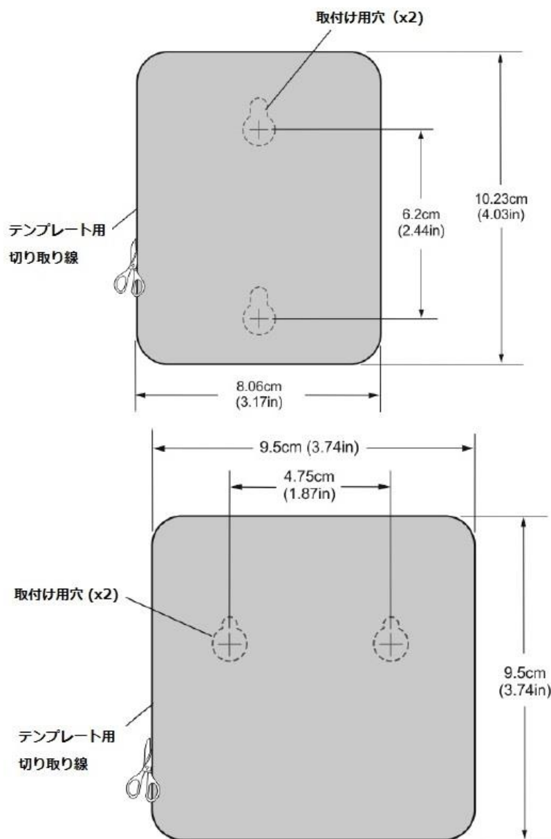
図11 取り付け穴位置図 (原寸ではありません)
