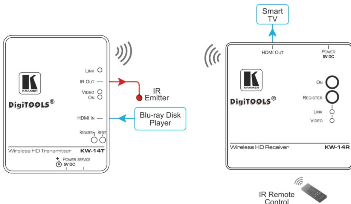
KW-14T、KW-14R 接続例
