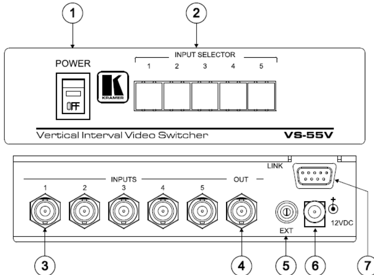
図 1 VS-55V フロント&リアパネルの機能説明
